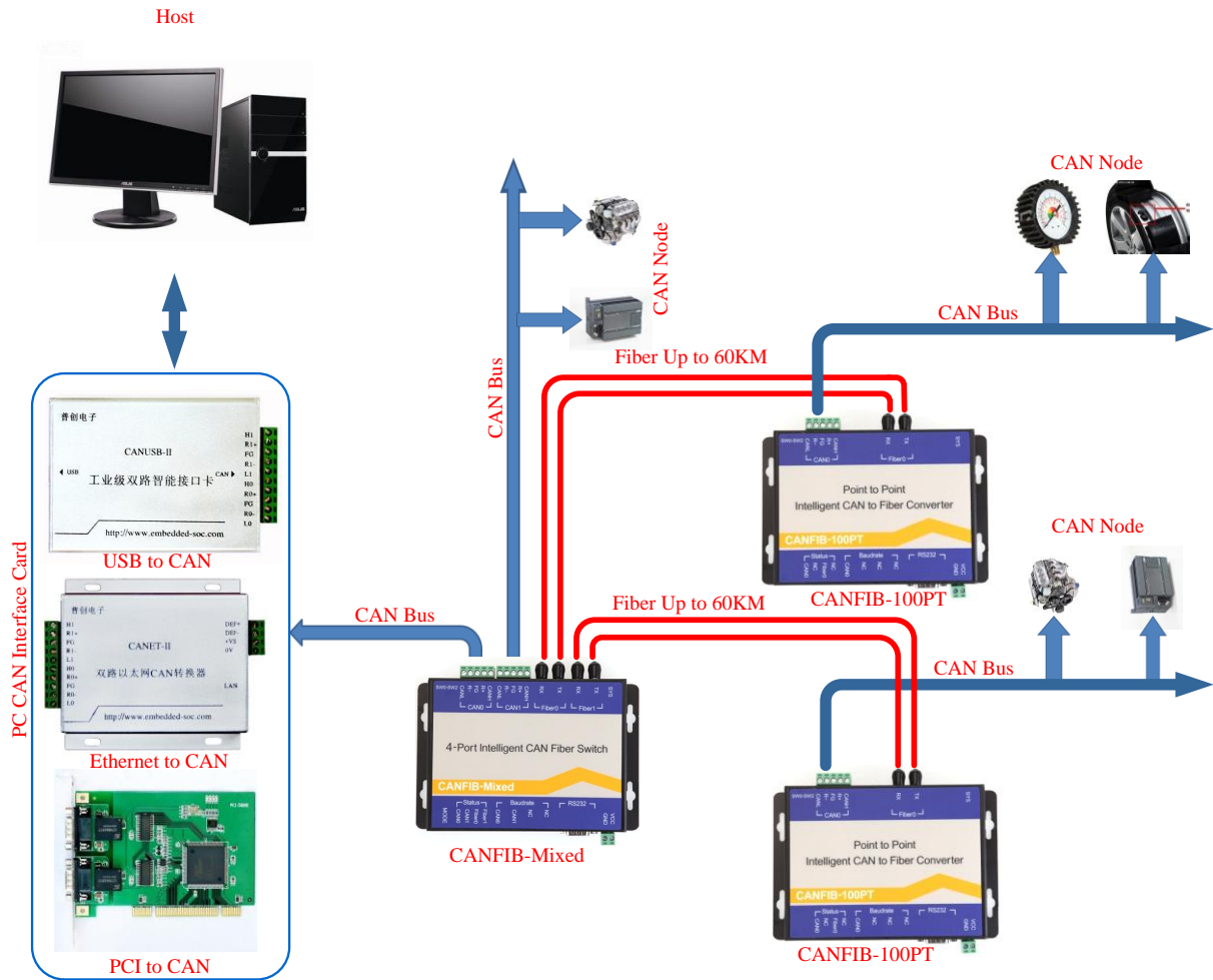
图 1-1-1 CANFIB-Mixed 智能CAN光纤交换机典型应用
