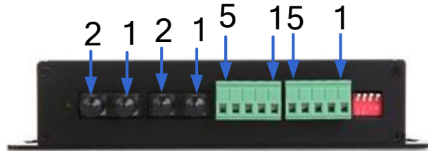
图2-2-2-1 CAN接线端子
