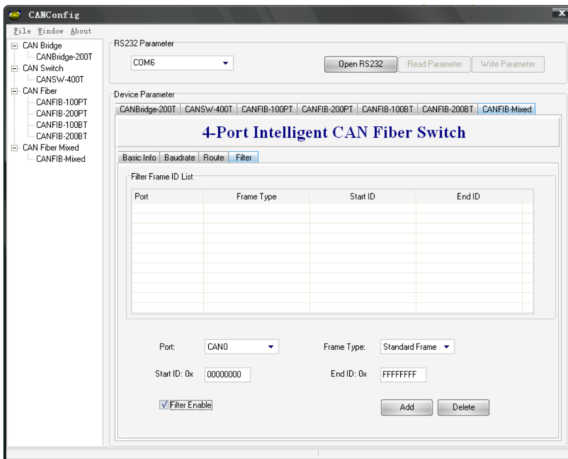
图 4-2-3-4-1 “Filter” 选项卡
